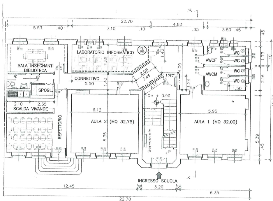
PIANTA PIANO RIALZATO
