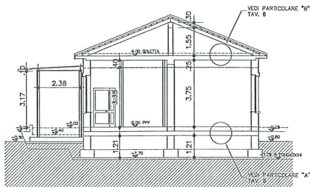
SEZIONE A-A
